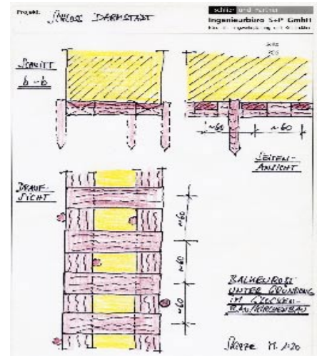
Skizze Gründungsrost
